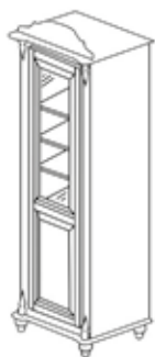
Шкаф книжный 1 ств. Арт. 3.26.01 (626x457x2110) Арт. 3.26.011 узк (626x330x1580)
