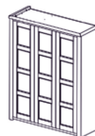
Шкаф 3-ств. (3.21.01) 1596x616x2000
