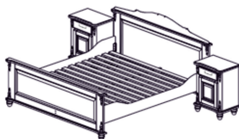
Двойная кровать Арт. 12.2.02 (1530x2134x1060/700) Арт. 12.2.03 (1730x2134x1060/700) Арт. 12.2.05 (1730x2134x1060/520) Арт. 12.2.04 (1930x2134x1060/700)
